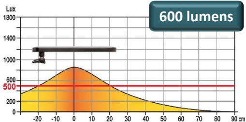
Curva LUX( 40 cm de la superficie de trabajo)
